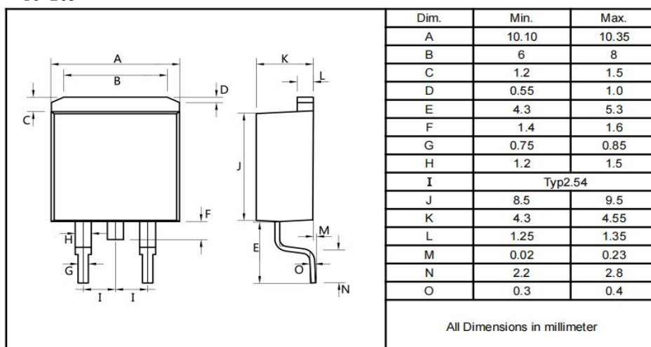
TO-263
